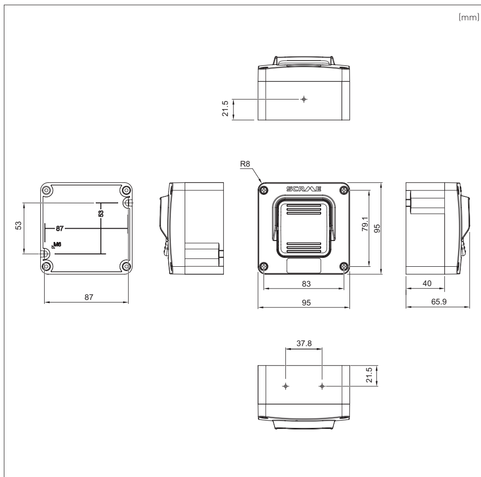
Figura 1 - Disegni tecnici
