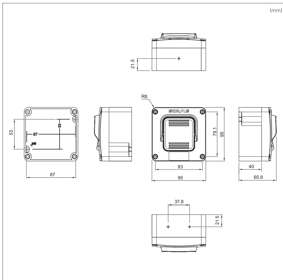
Figura 1 - Desenhos técnicos
