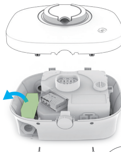
TX10 Tornillo Torx M3x16mm x2
